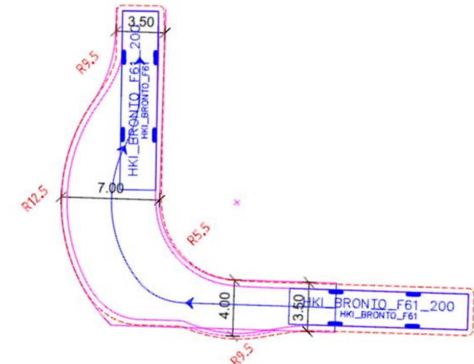
Kuva 1. Nostolavayksikön ajouramalli.
